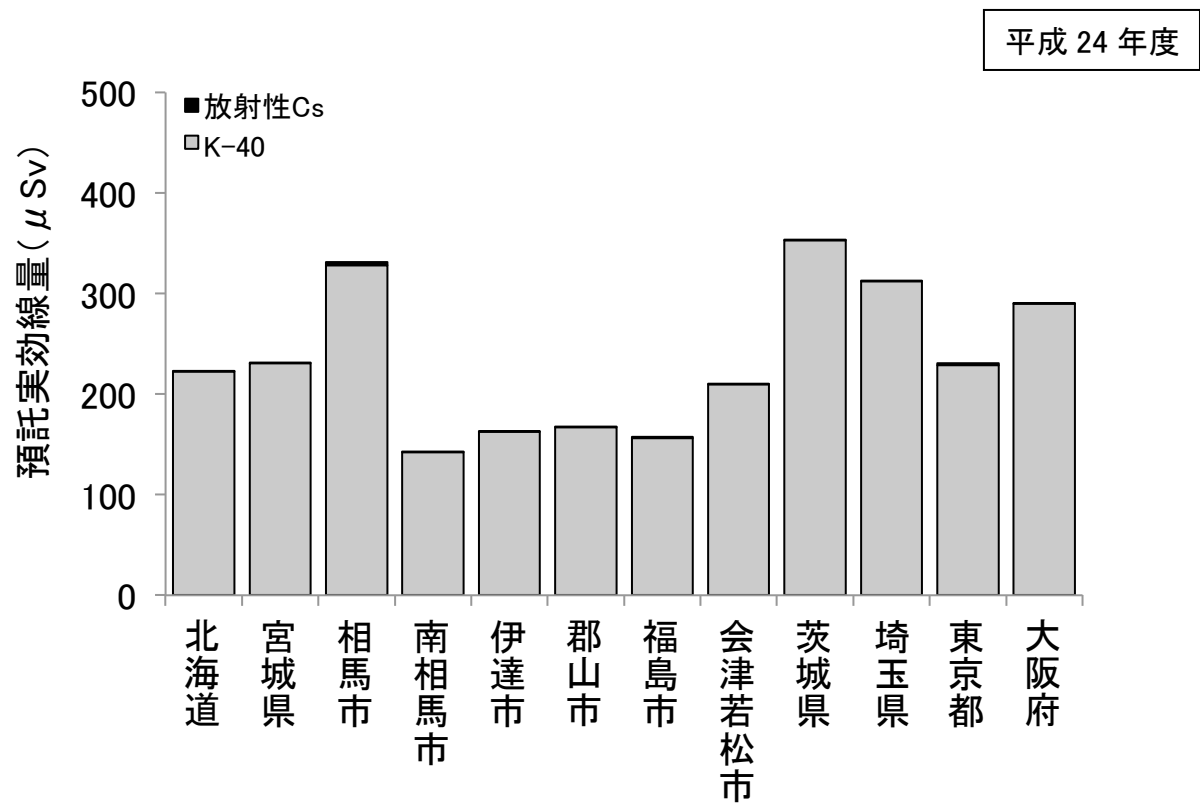
図 8. 陰膳試料による放射性 Cs と 40 K の預託実効線量の地域別平均値(幼児)
