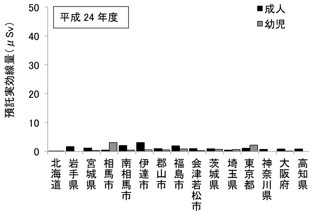
図 6. 陰膳試料による放射性 Cs の預託実効線量の地域別平均値
