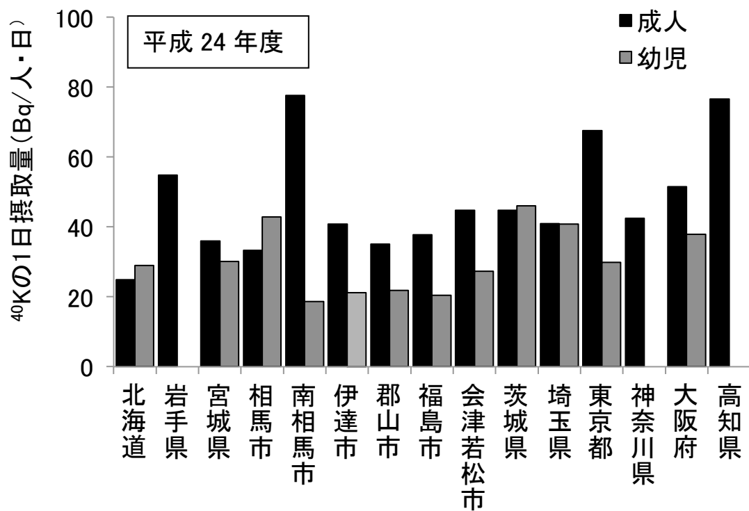
図 5. 陰膳試料による ^{40}\text{K} の 1 日摂取量の地域別平均値
