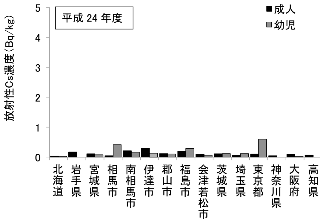
図 2. 陰膳試料中の放射性 Cs 濃度の地域別平均値
