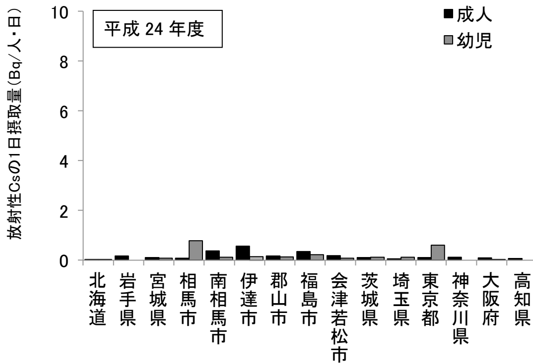
図 4. 陰膳試料による放射性 Cs の 1 日摂取量の地域別平均値
