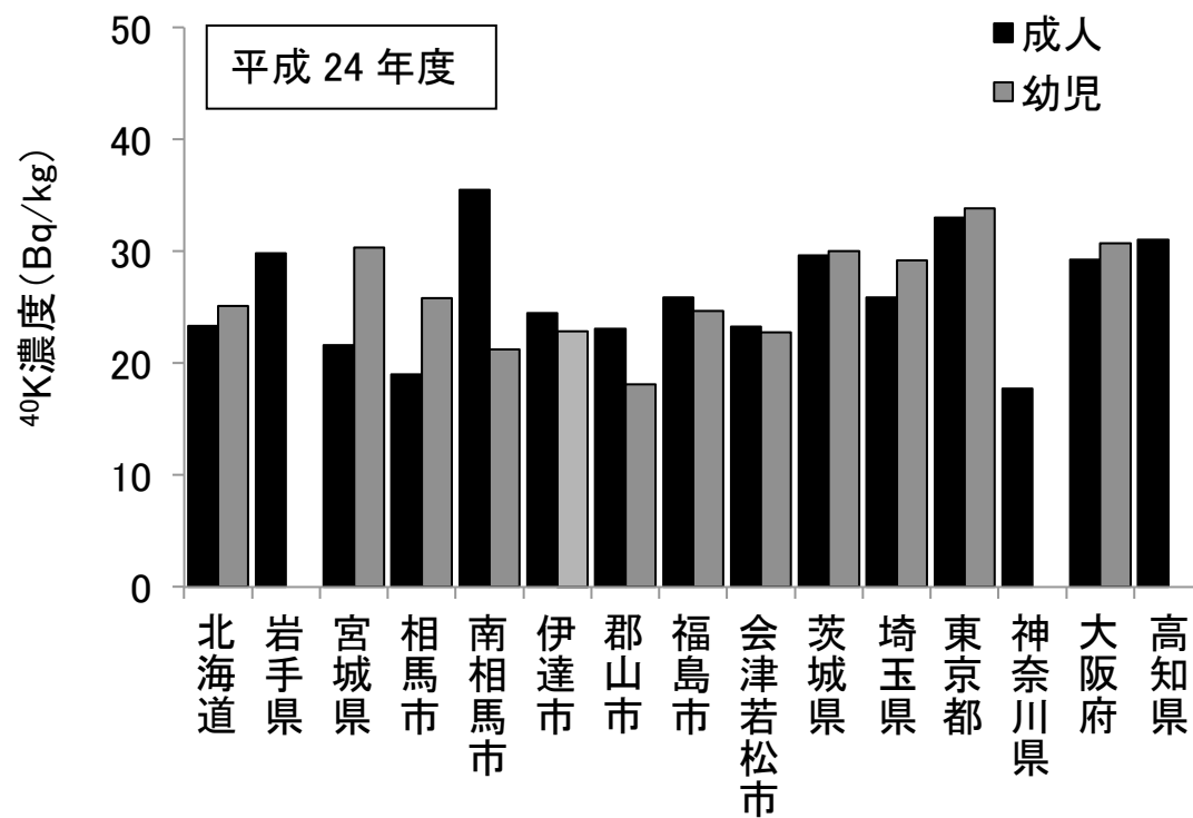
図 3. 陰膳試料中の ^{40}\text{K} 濃度の地域別平均値
