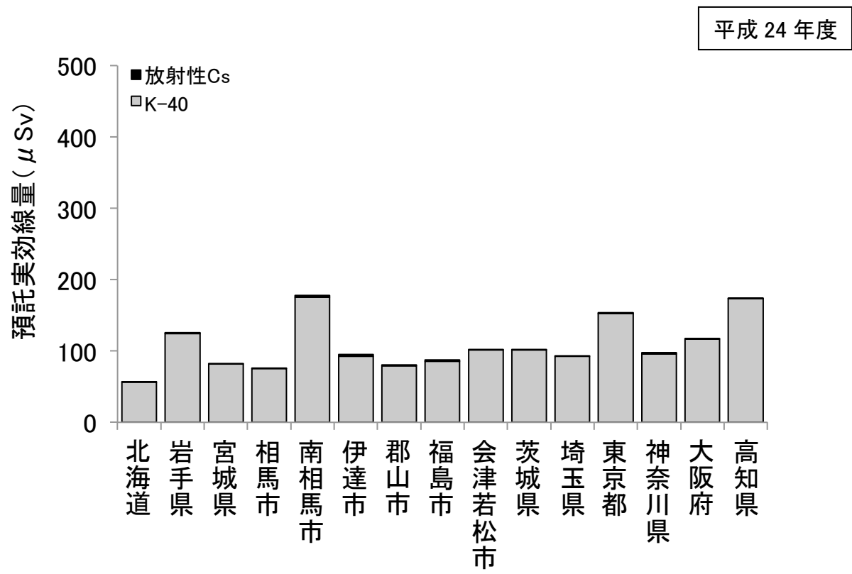
図 7. 陰膳試料による放射性 Cs と 40 K の預託実効線量の地域別平均値(成人)
