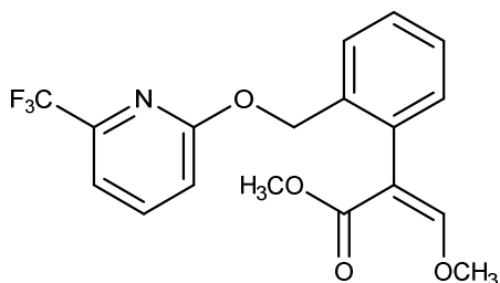
代謝物 B
