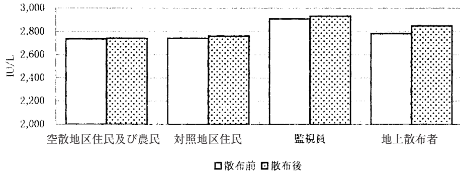
図8 空中散布後のコリンエステラーゼ活性
