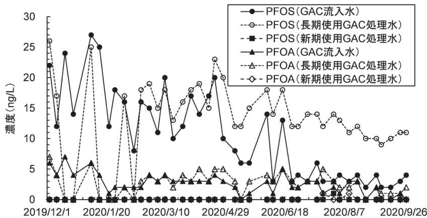
図1 GAC処理によるPFOS, PFOA濃度の推移(対象水はオゾン処理水;長期使用GACは2016年度より使用;長期使用GAC処理水は2019年12月16, 23日, 2020年1月14～27日, 2月20日が, 新規使用GAC処理水は2020年7月7日が未測定)[40]
