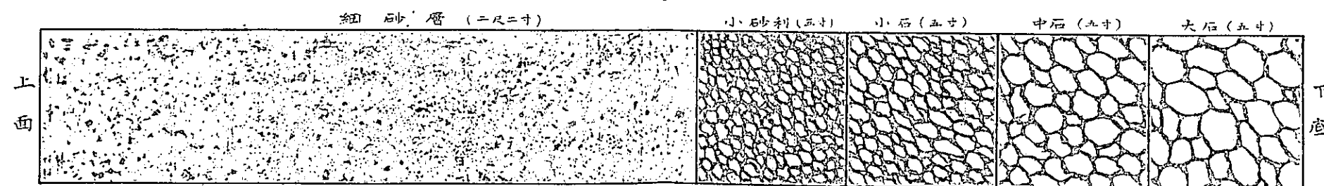
七市水道，濾床細砂層，濾砂混合比較（百分比例）
