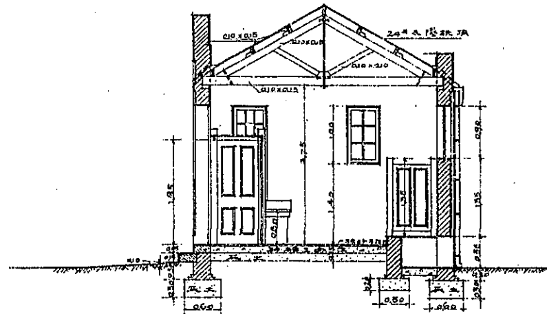
橫剖面圖
