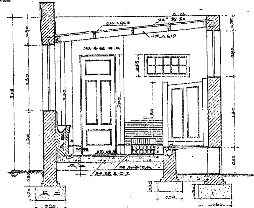
侧面图(一)
