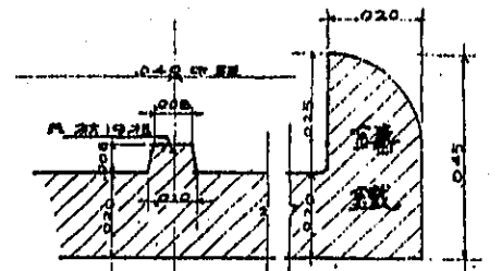
合面平 (B)
