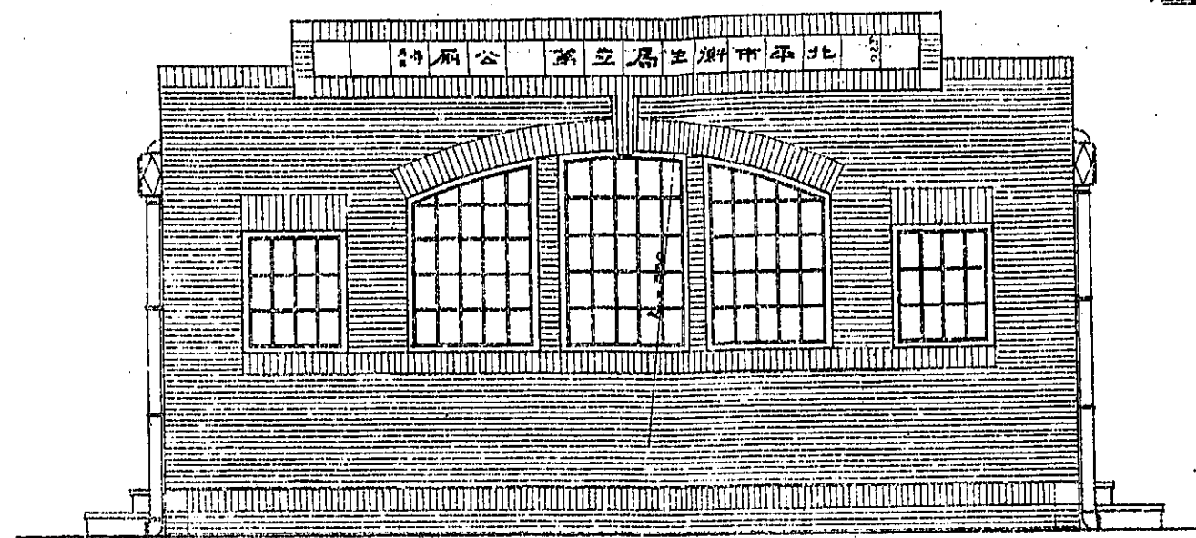
正面图
