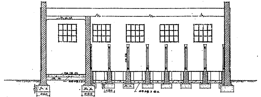
縱剖面圖
