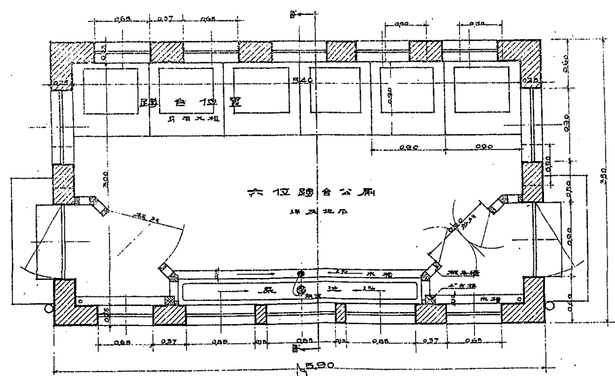
平面图
