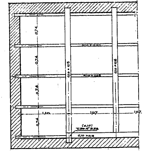
平面图(二)
