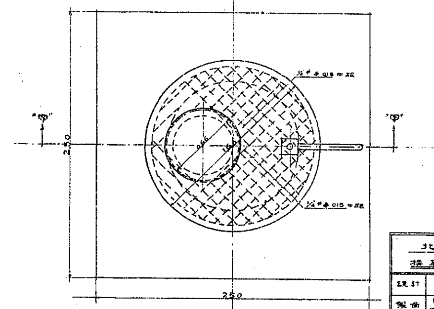
平面圖
