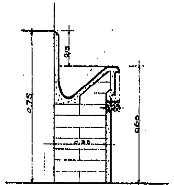
A-B 剖面圖
