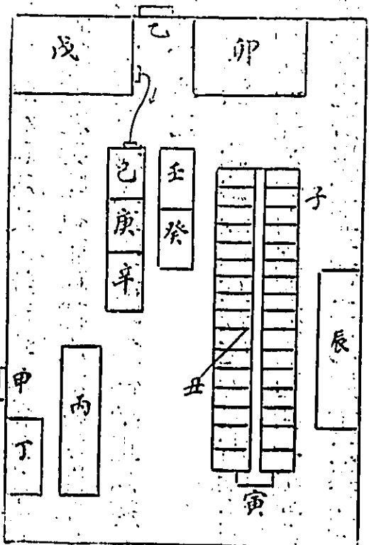
式圖造構舍離隔
